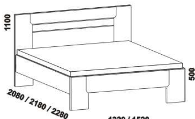
1320 / 1520 1720 / 1920 / 2120 postel SAFIRA, vykrojené nohy předního čela 120, 140 x 200, 210, 220 160, 180, 200 x 200, 210, 220
