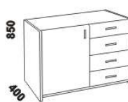
850 400 1010 komoda 1dveřová 4zásuvková dveře L nebo P
